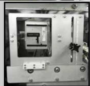
Montiert auf einer vertikalen Verpackungsmaschine (Schlauchbeutelmaschine)
